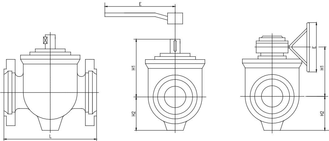
Dimensions and Weights 尺寸及重量 (Class600 ~ Class1500)
