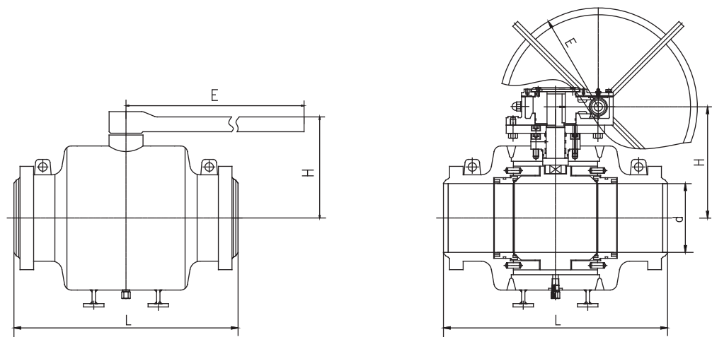
Dimensions and Weights 尺寸及重量 (Class150 ~ Class300)
